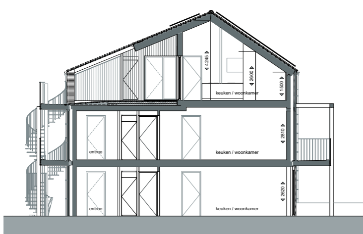
Doorsnede A-A
