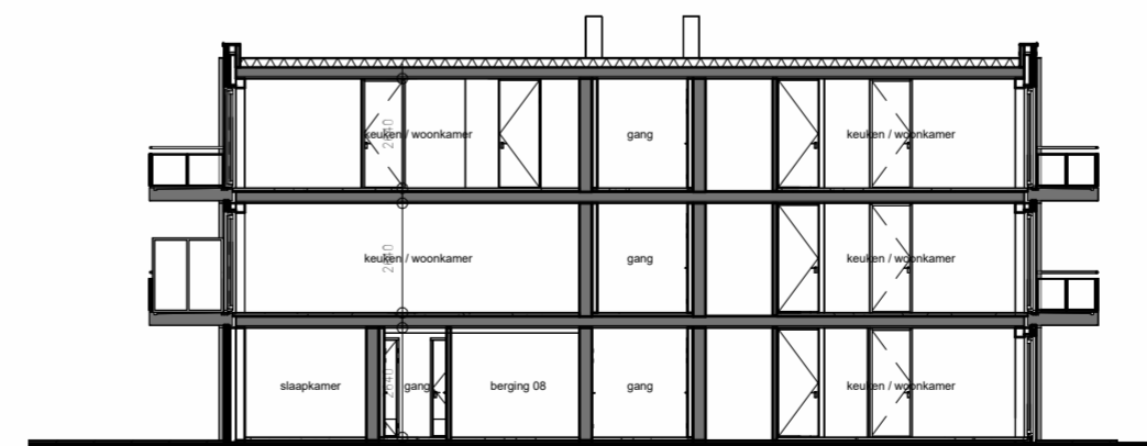
Doorsnede B-B
