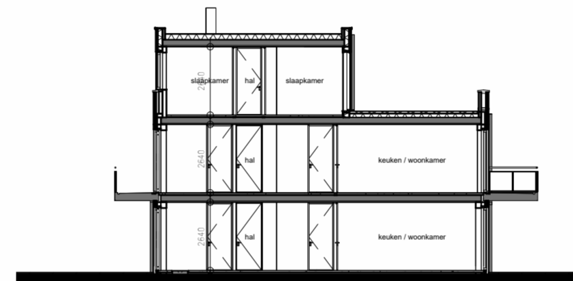
Doorsnede A-A
